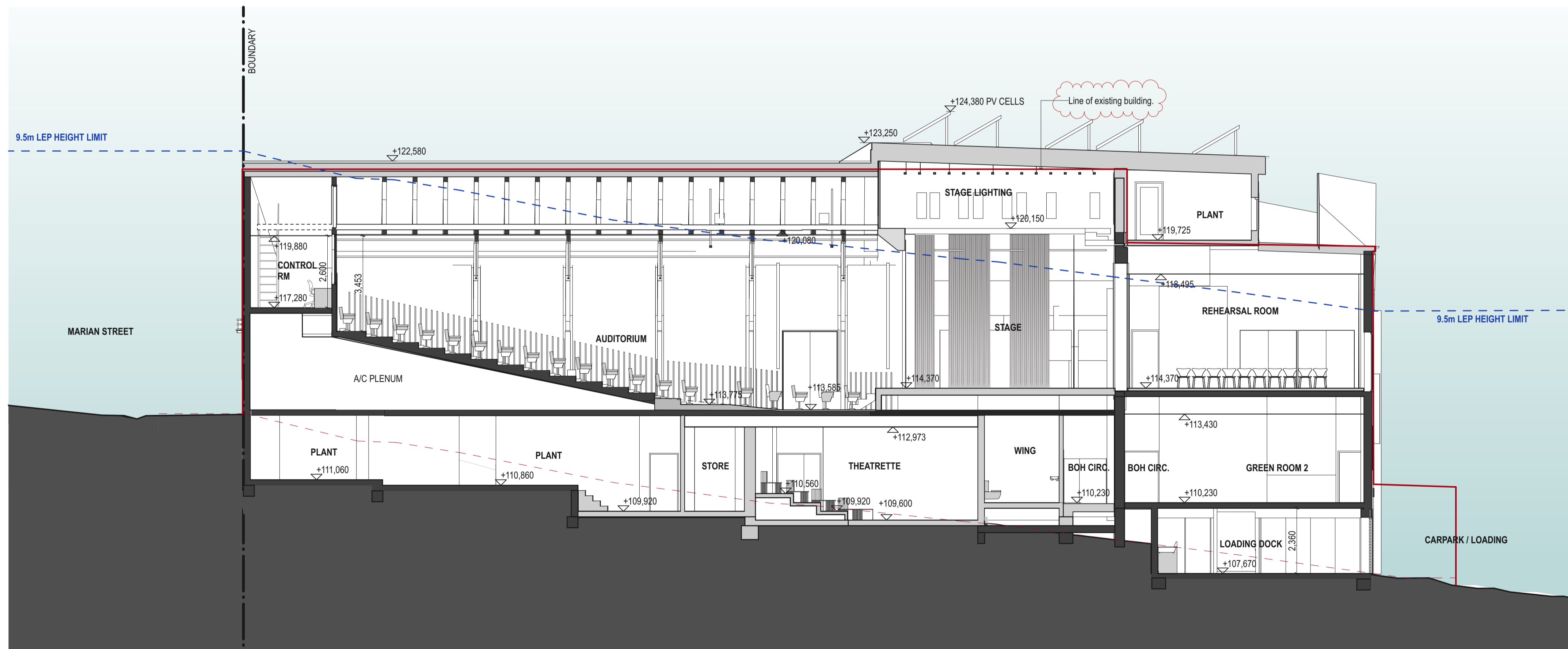
2 LONGITUDINAL SECTION - 2 1:100
