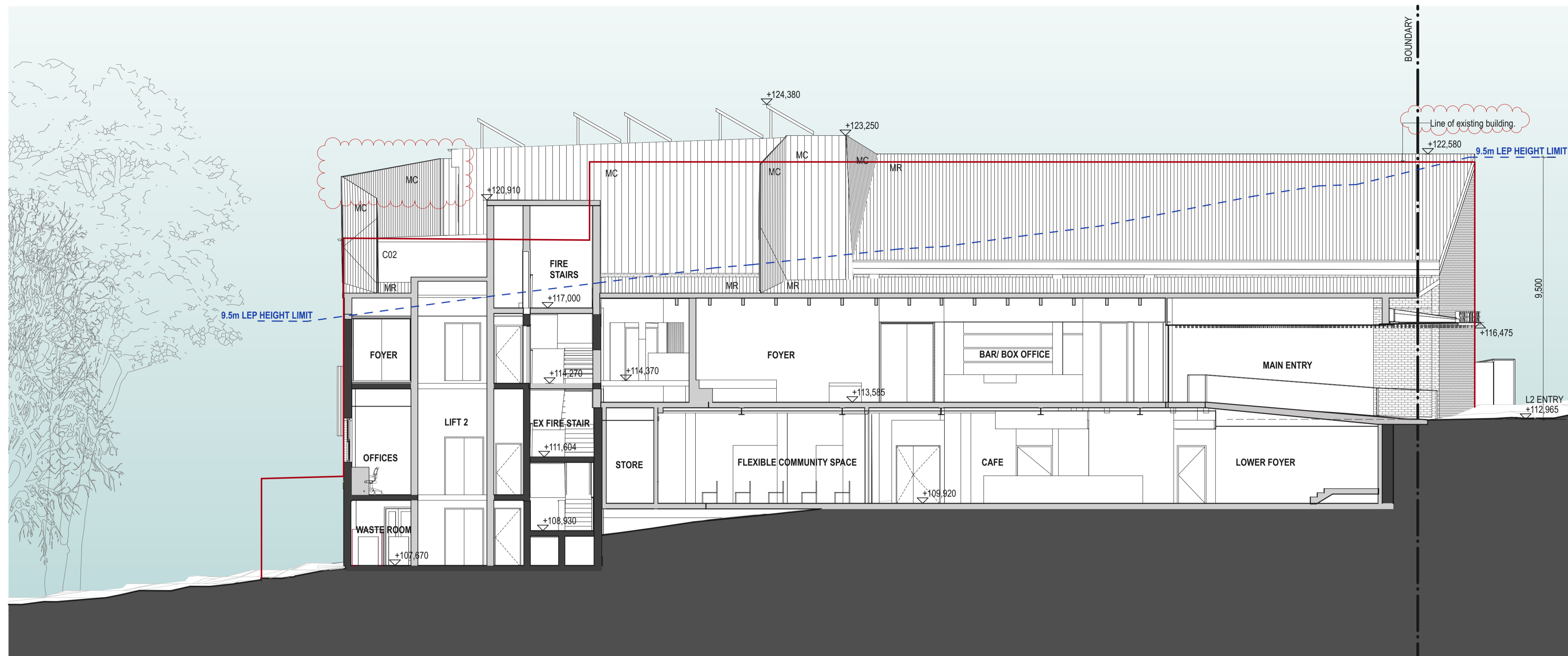
1 LONGITUDINAL SECTION - 1 1:100
